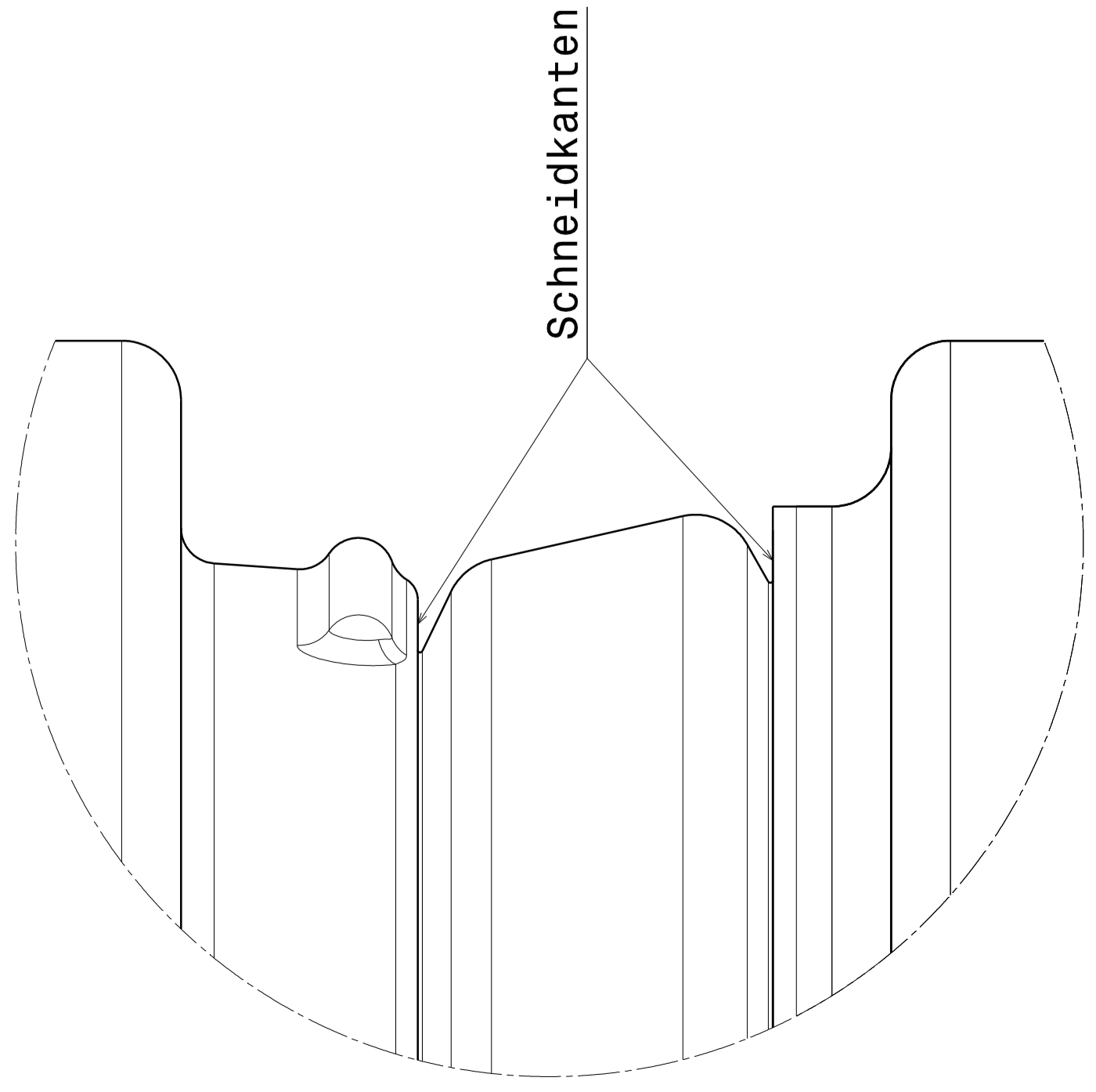
Einzelheit A M 2:1
