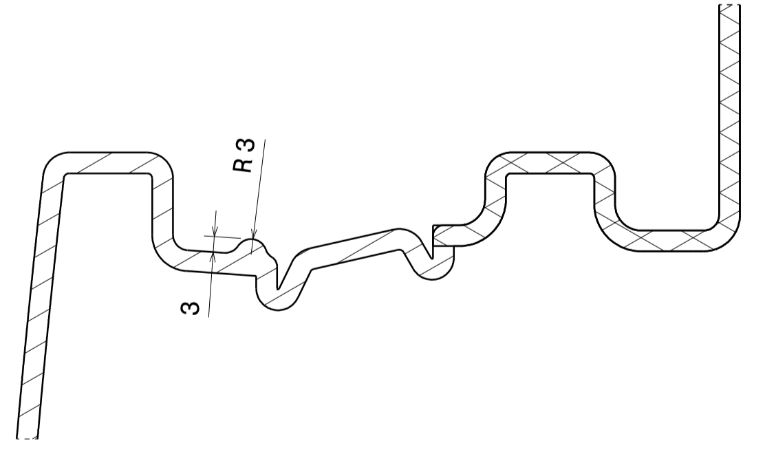
Schnitt B-B M 1:1
