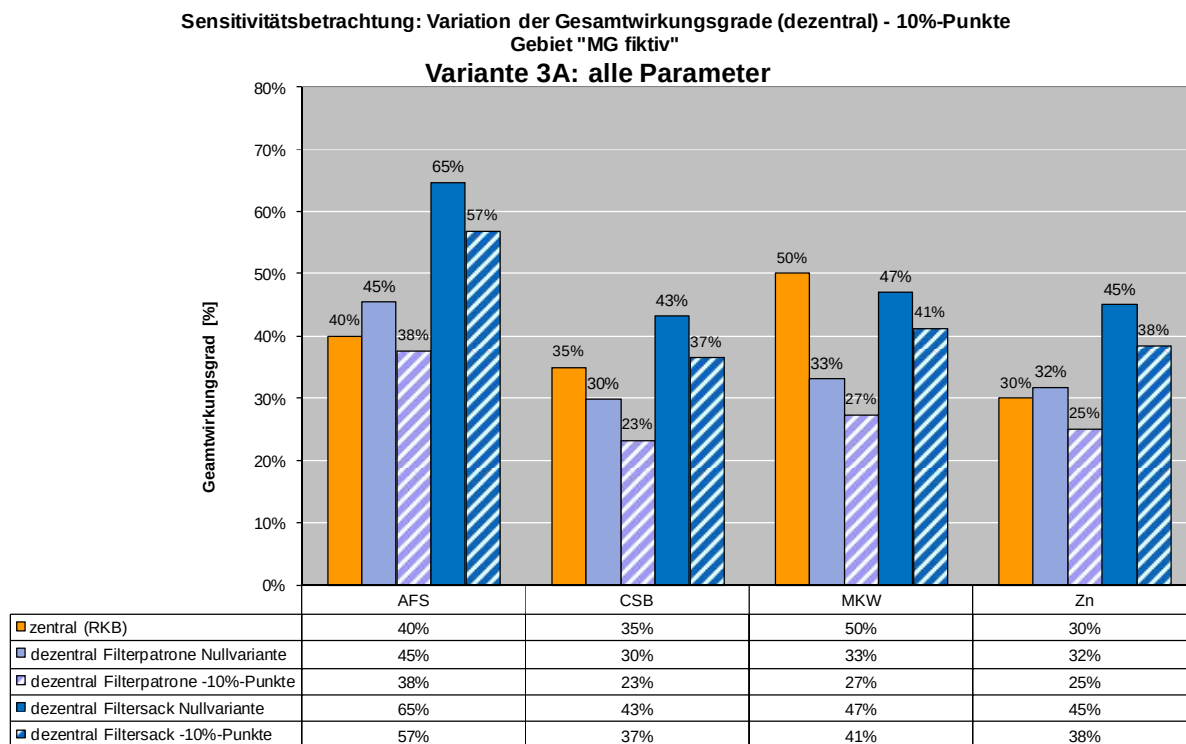
Abbildung 71: Variante 3 (Variation der Gesamtwirkungsgrade dezentral): alle Parameter, MG fiktiv
