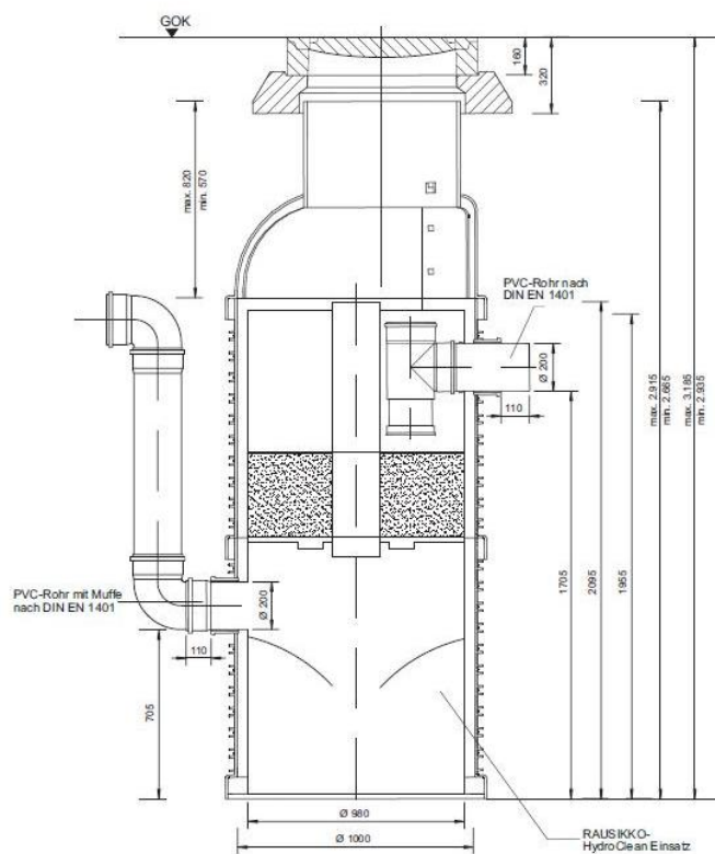
Abbildung 57: 3P Hydrosystem Einbauskizze
